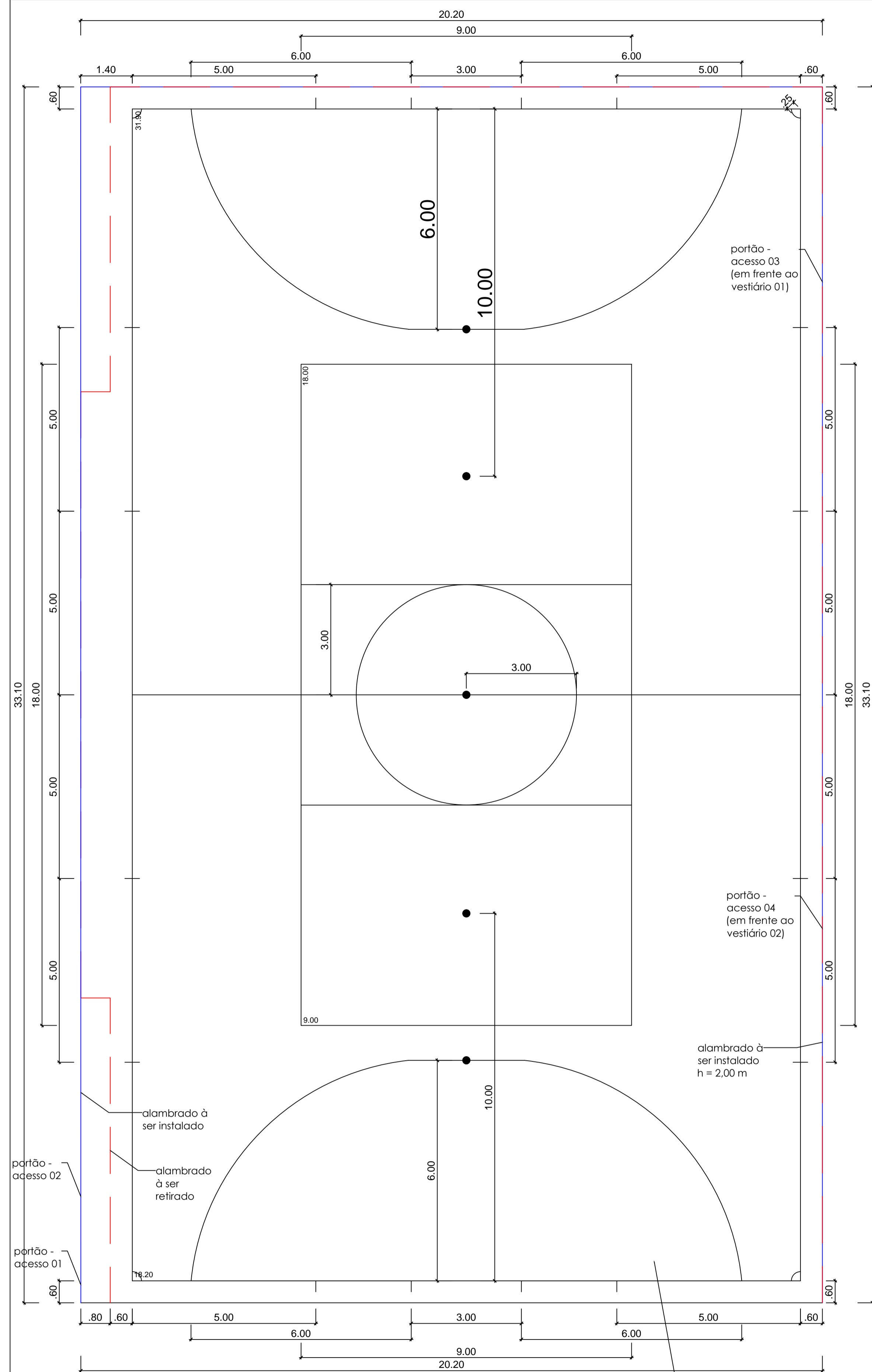
PROJETO ARQUITETÔNICO - Reforma de Quadra Escala 1:75 Área: 668,62 m 2
