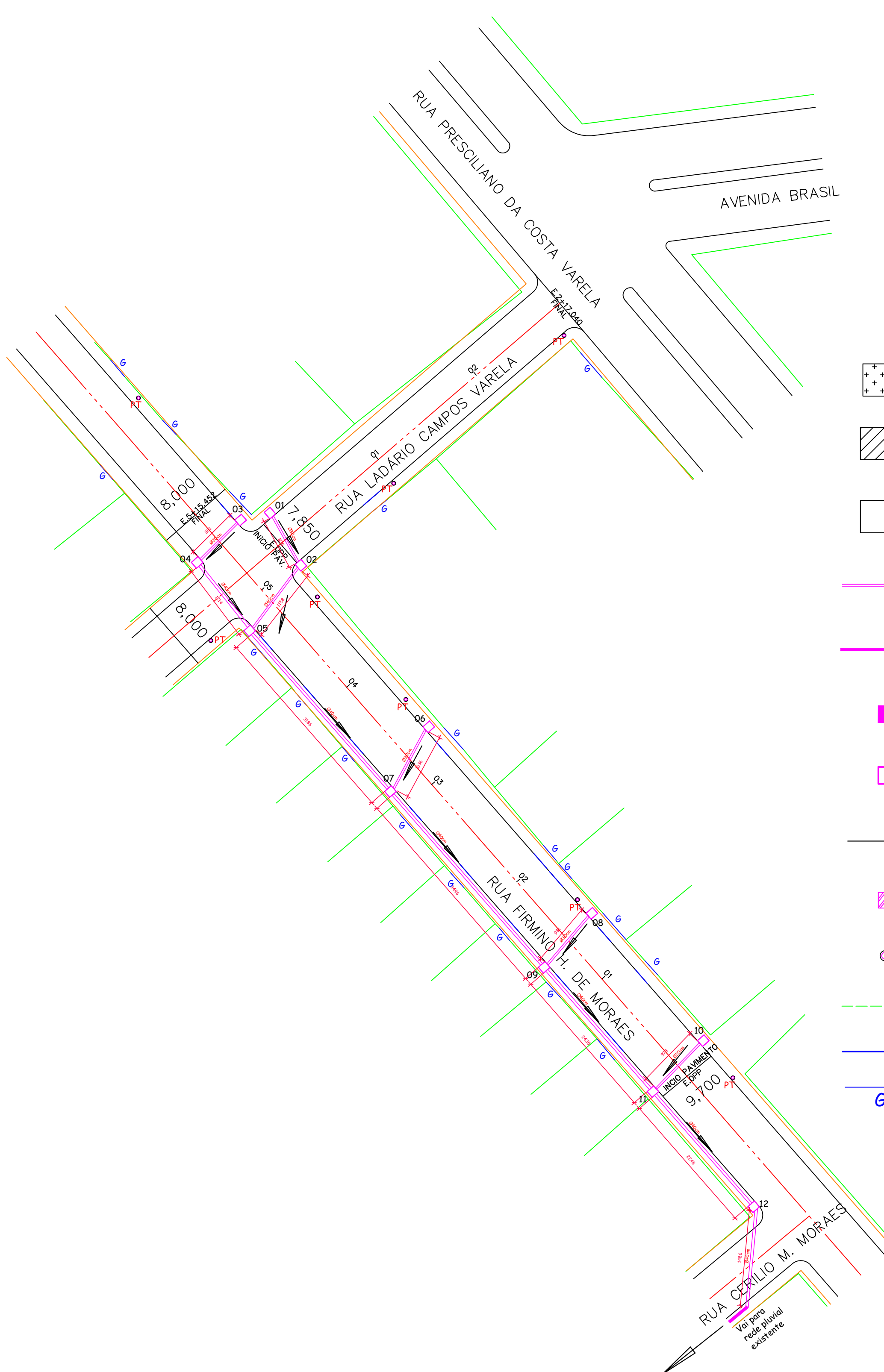
Rede Pluvial
